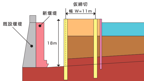
補強断面図
