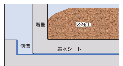
底部詳細図
